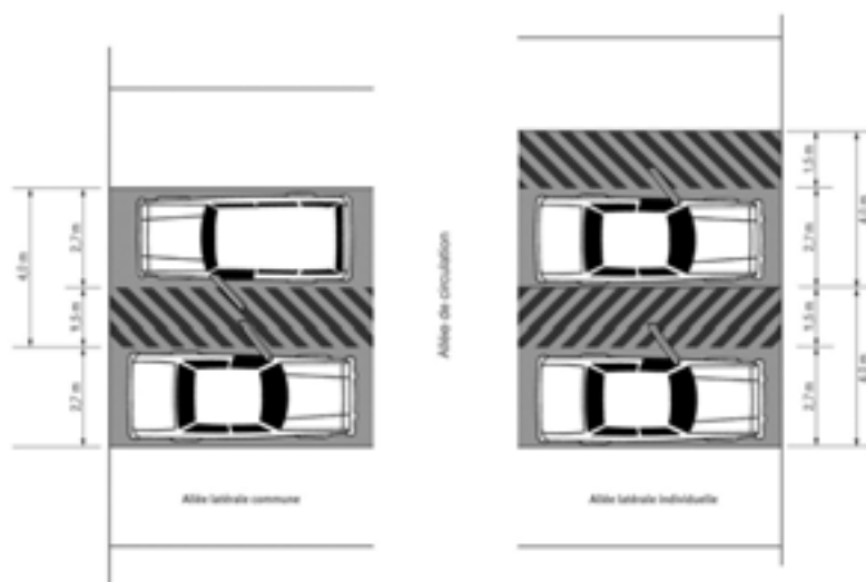
Illustration 3. Cases de stationnement réservées aux personnes handicapées avec allée latérale commune ou individuelle.
