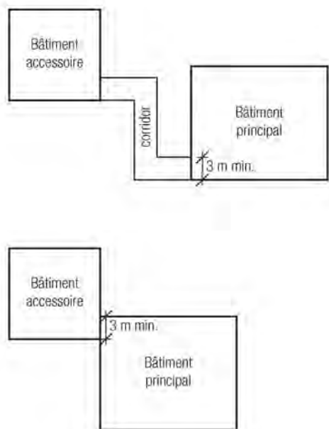
Illustration 10. Bâtiment accessoire attaché
