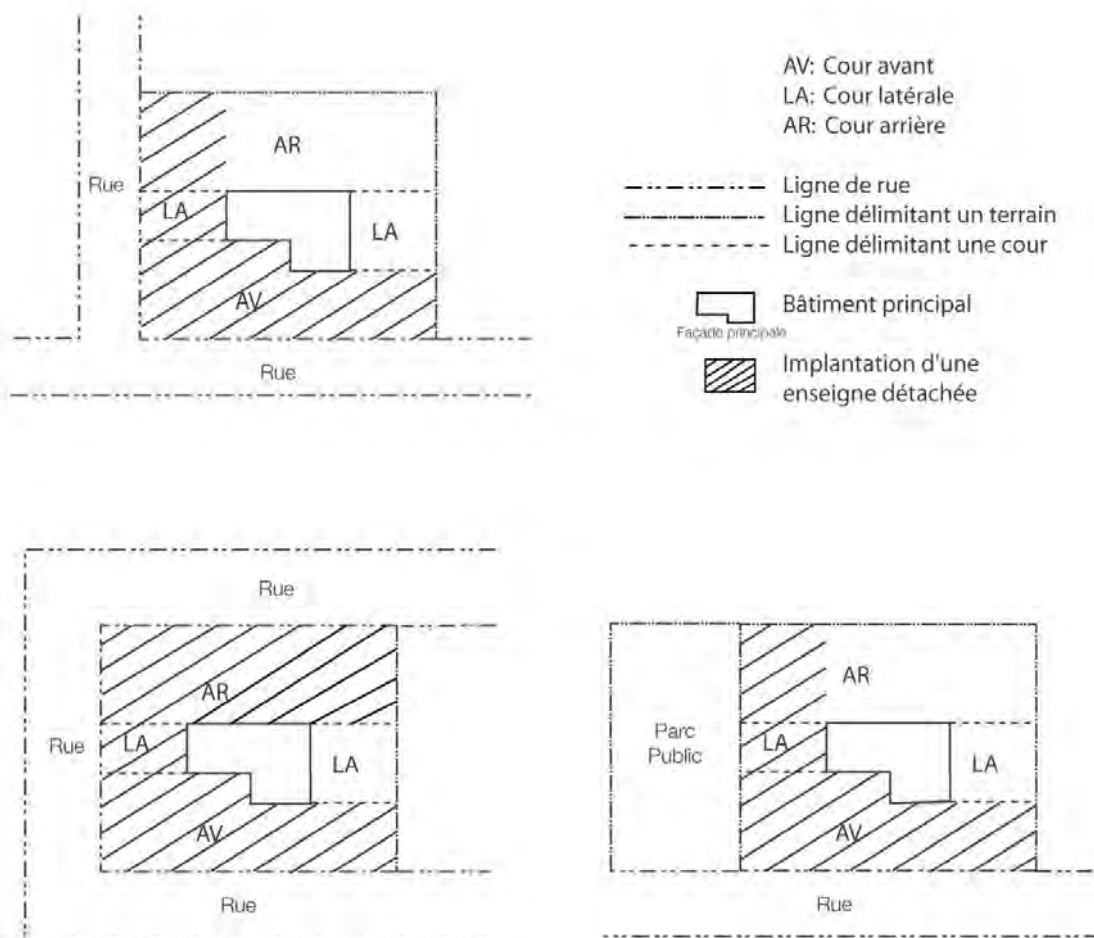
Illustration 7. Implantation d'une enseigne détachée
