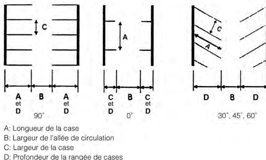
Illustration 2. Dimensions des cases de stationnement et des allées de circulation.
