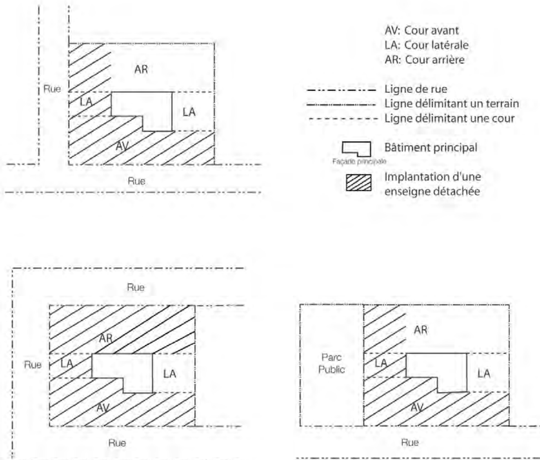
Illustration 6. Implantation d'une enseigne détachée
